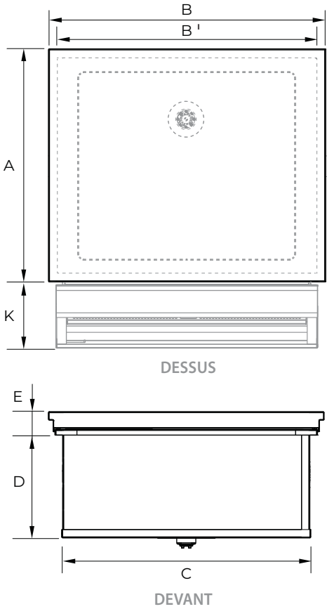
Dimensions du bâti pouces (mm)
