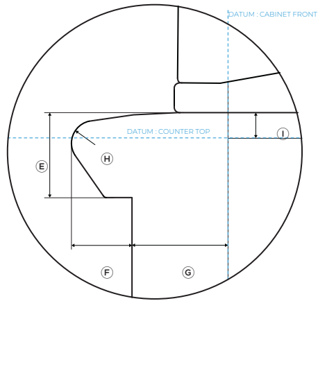
VUE DÉTAILLÉE - BARBECUE NEZ DE BŒUF
